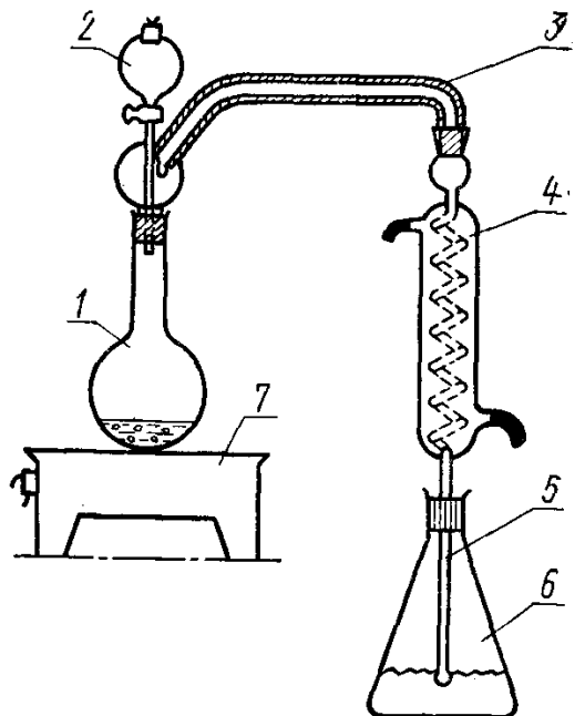
1—дистилляционная колба вместимостью 100 мл; 2—насадка с капельной воронкой; 3—дефлегматор с соединительной трубкой; 4—змеевиковый холодильник; 5—барбатер; 6—пробирка-приемник; 7—электроплитка.
