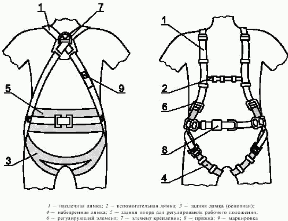
Рисунок 1 — Пример исполнения страховочной привязи
