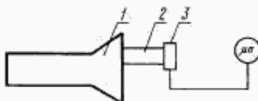
1 — электронно-лучевой прибор (ЭЛП, ЦЭЛП); 2 — тубус; 3 — фотоэлемент
