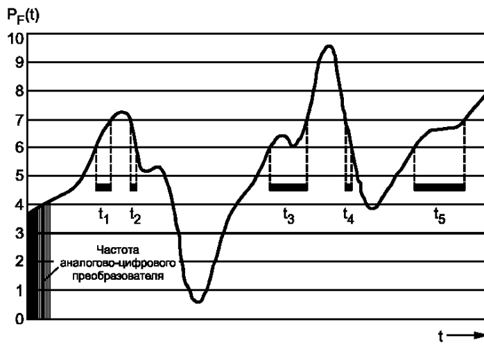
Рисунок 2а — Уровень фликера как функция времени
